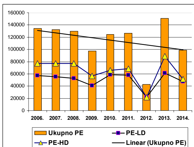
SLIKA 1. Kretanje proizvodnje polietilena u fabrici HIP-PETROHEMIJA u Pančevu (manja proizvodnja u 2012. posledica je remonta i rekonstrukcije fabrike)
